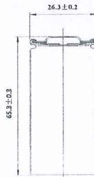
图 1 电芯外观尺寸
