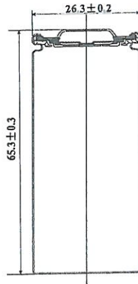
图 1 电芯外观尺寸
